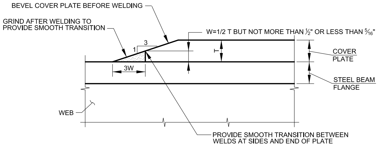
ELEVATION
